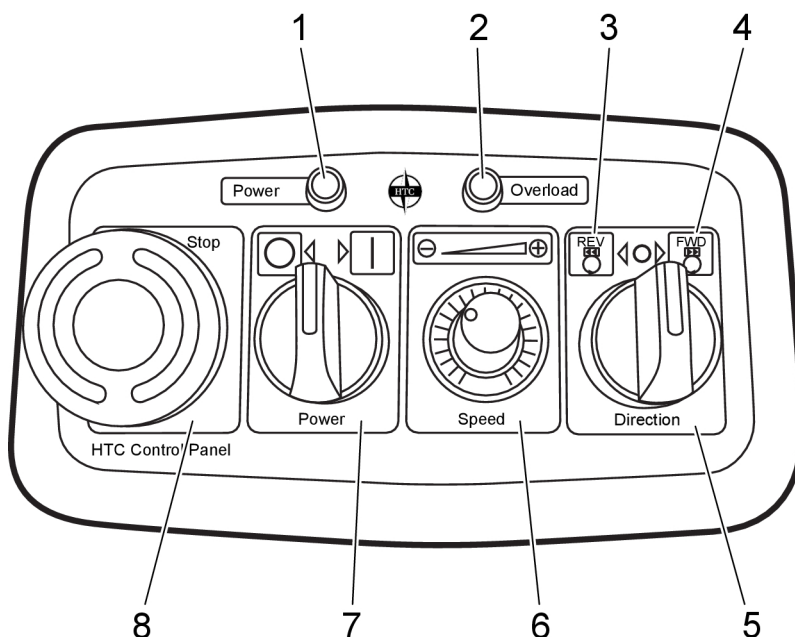
Figura 3-3. Panel de mando
